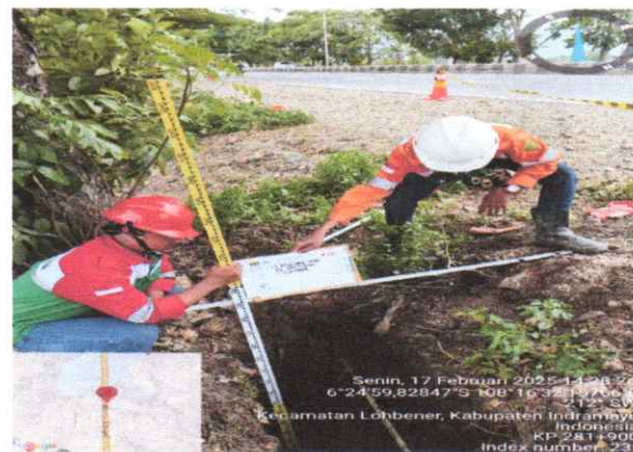
Judul Foto penukuran kedalam, lebar dan panjang pit. Tanggal 17 Februari 2025 Loc KP 282+900
